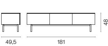
CS6211-3
